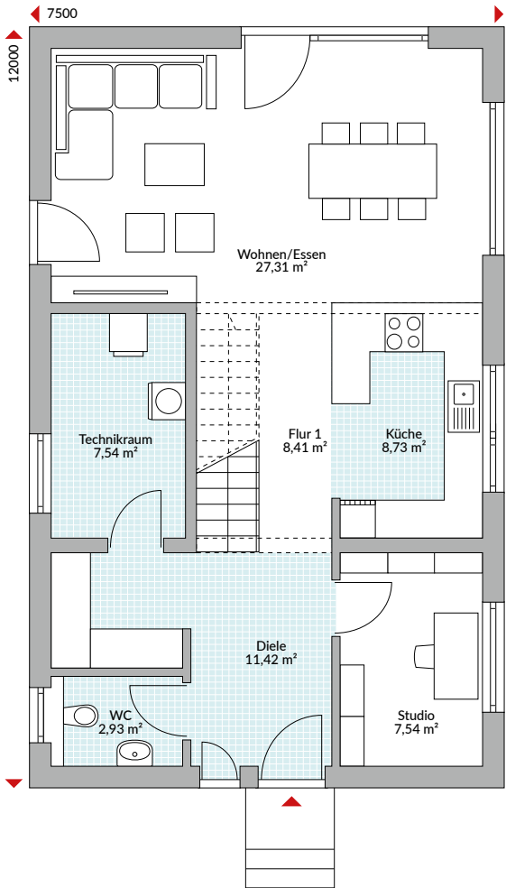
Erdgeschoss 73,88 m 2
